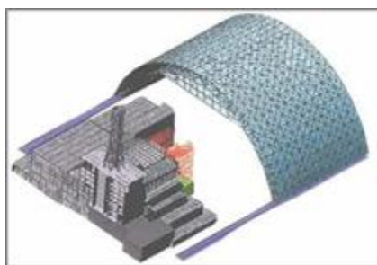
Конструкція конфайнменту Чорнобильської АЕС
